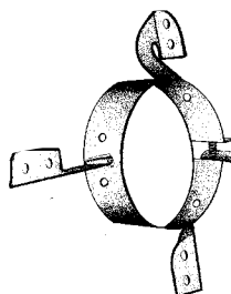
92-A8556 9" Bolt Circle
